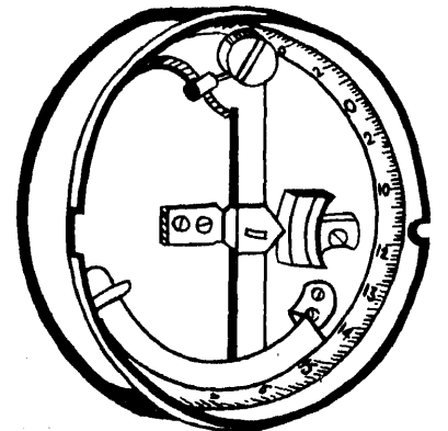
Clinometer : कलमापक
